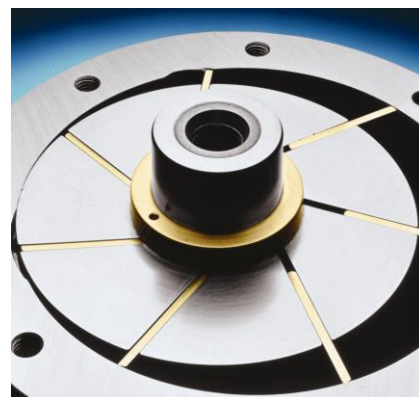
Figure n° 1 - Technologie rotative à palettes
