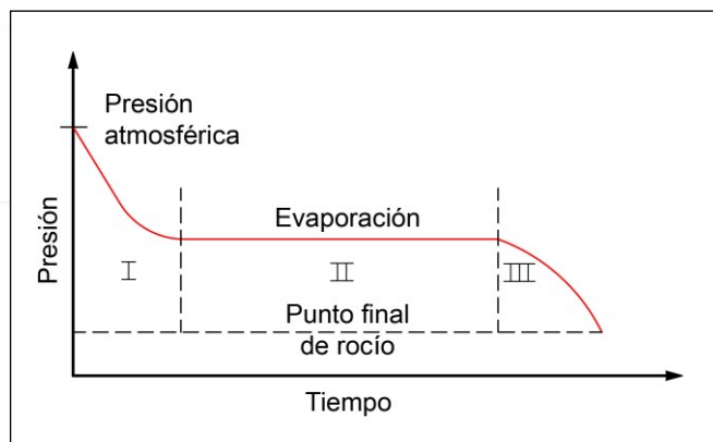
Proceso de secado de cañerías con vacío
